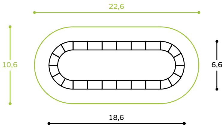
Altura libre de caída / Área de seguridad / Free fall height / Safety area Hauter libre de chute / Zone de sécurité / Freie Fallhöhe / Sicherheits- Schutzbereich
